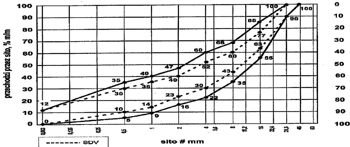
Rysunek 1. Uziarnienie mieszanki niezwiązanej 0/31,5 do podbudowy pomocniczej
