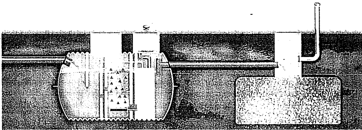
Rys.2 Schemat rozwiązania oczyszczalni z zastosowaniem studni chłonnych
